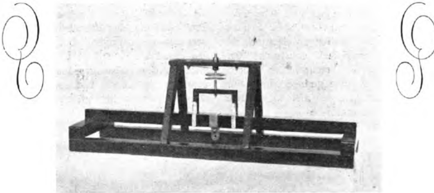
Het gewicht van een paardenhaar, die op de ijzerstaaf gelegd wordt is toereikend om door de Ultra-Micrometer vastgesteld te worden
