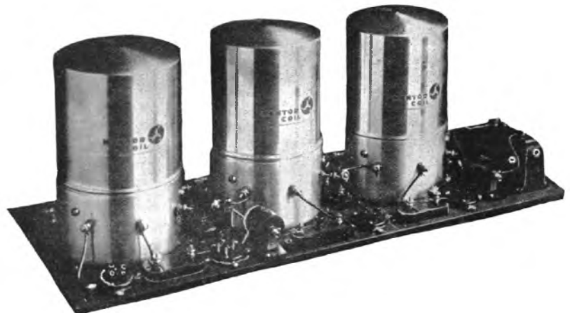
Het binnenwerk van R.W.'s 1929 Solodyne
