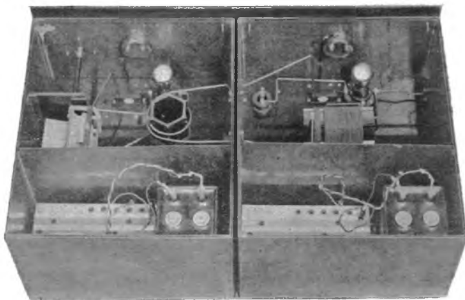
Binnen-aanzicht van den Electro-Ultramicrometer
