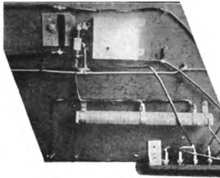
De aansluiting van den Electrad-2000 ohm-aftakweerstand, welke automatisch voor de vereischte roosterspanningen zorgdraagt
