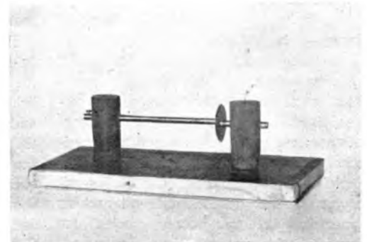
Een geringe verwarming van den metaal-staaf (links), een aanraking met de hand, zal een verandering in den zwevingstoon teweeg brengen
