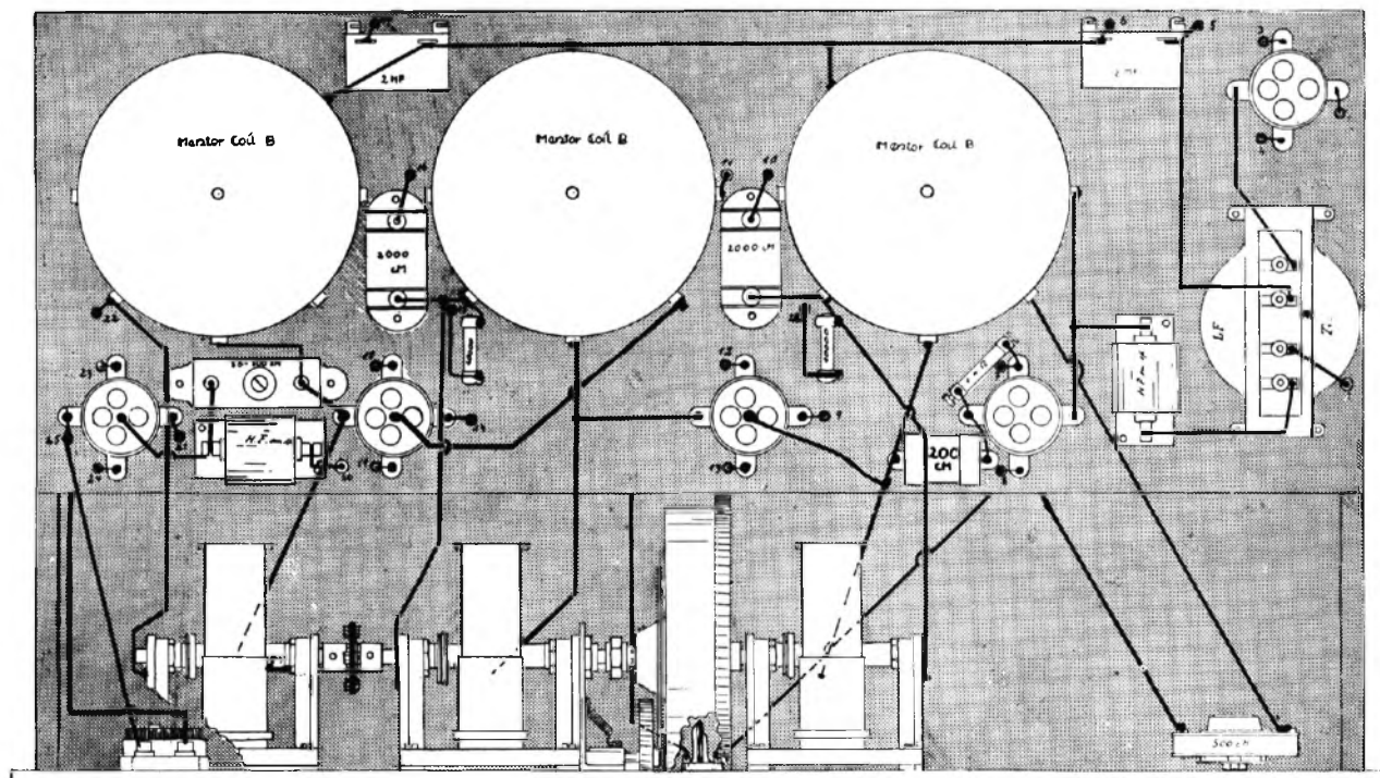
Werkteekening op een derde van de ware grootte, een overzicht gevende van de plaatsing der onderdelen op de bovenplank en van den loop der verschillende verbindingsdraden tusschen de diverse onderdeelen op en onder de triplex-plaat. De cijfers bij sommige draden correspondeeren met die van draden onder de plank (zie het schema op blz. 29), zij duiden aan dat de genummerde verbinding doorloopt ook aan de onderzijde
